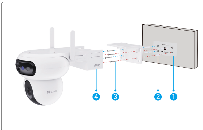
圖 2 壁掛式安裝
