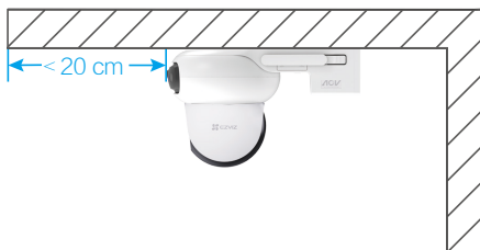
圖 2 壁掛式安裝
